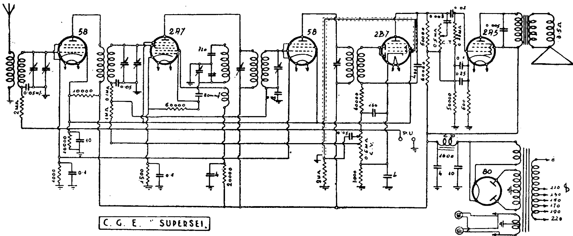
COMPAGNIA GENERALE DI ELETTRICITÀ. — Mod. « Supersei consolle » e Mod. « Supersei radiofonografo ». - Produzione 1933. - Media frequenza: 175 kc.
